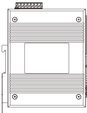
右侧视图
