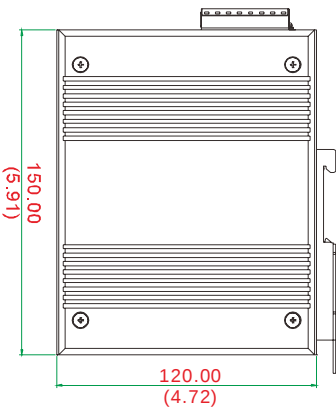
左侧视图
