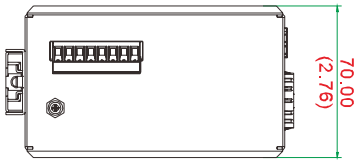
顶视图
